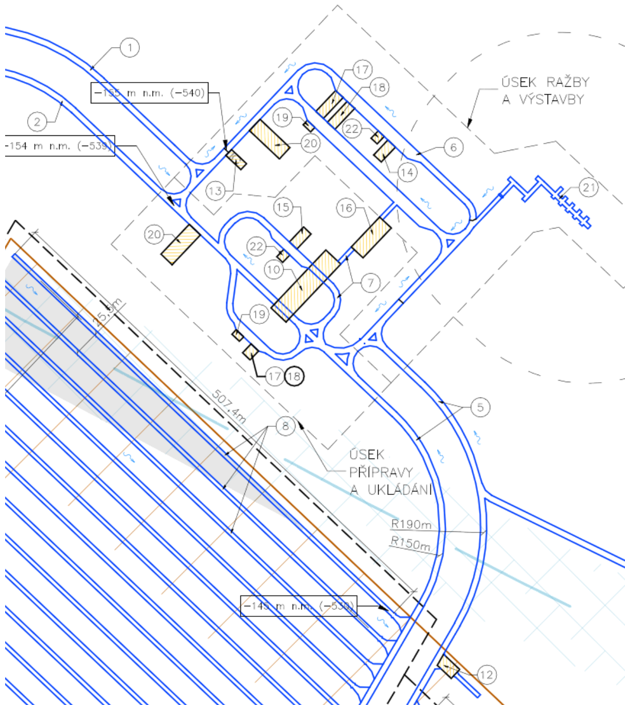
Obr. 59 – Schéma technického zázemí - D2
