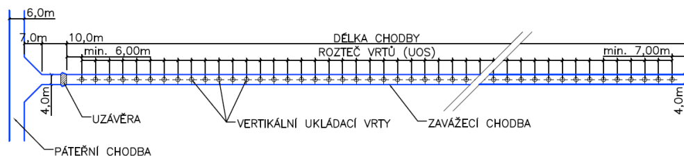
Obr. 53 – Schéma vertikálního ukládání, převládající konvenční ražba (D2)
