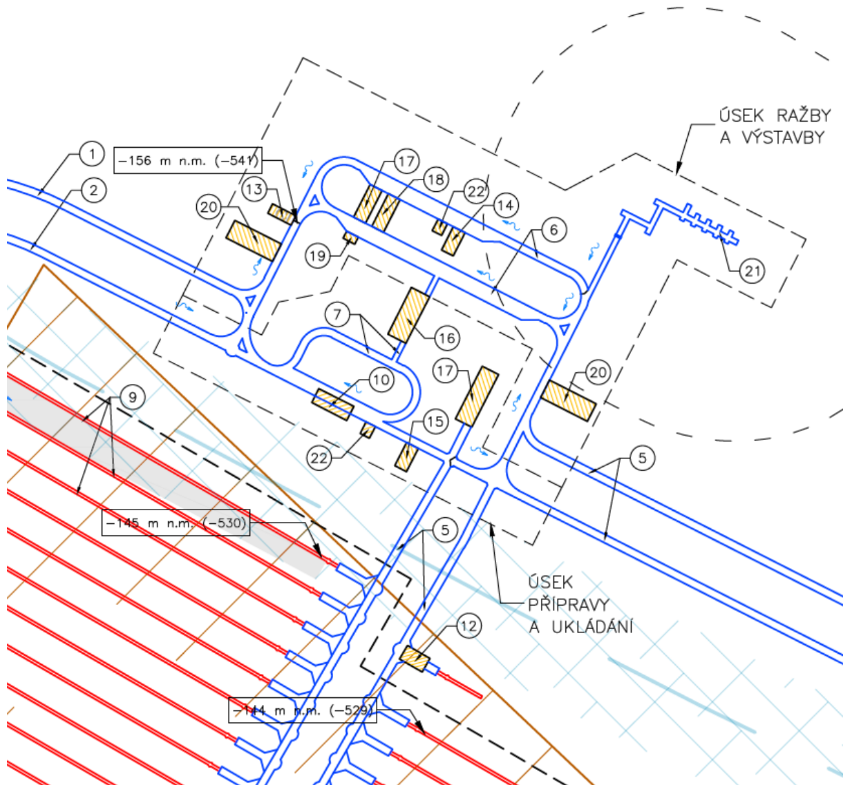
Obr. 60 – Schéma technického zázemí - D4
