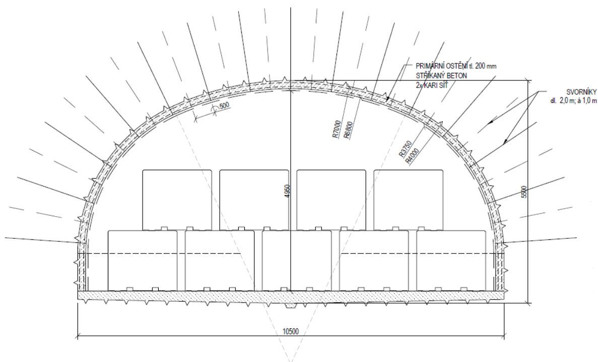
Obr. 90 – Příčný řez komorou pro ukládání RAO
