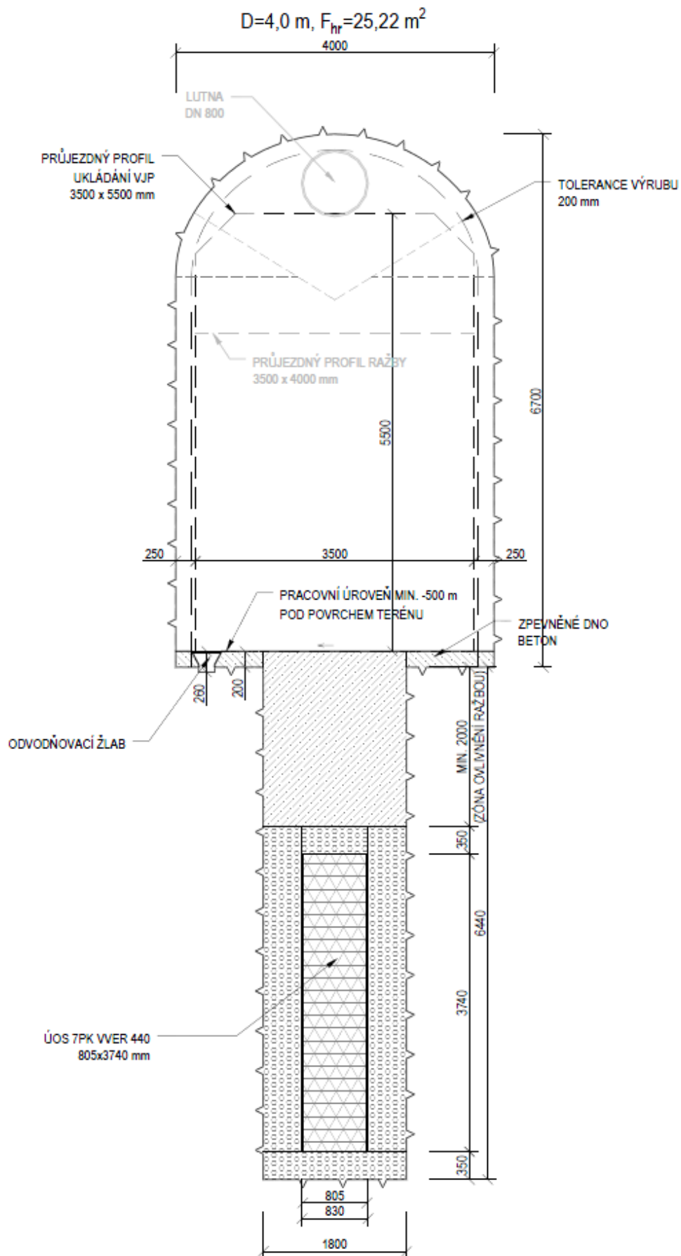
Obr. 83 - Vertikální uložení UOS (VVER 440) z ukládací chodby ražené konvenčně - D2
