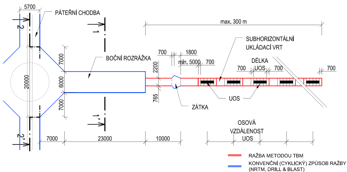
Obr. 86 – Půdorysné schéma ukládání – varianta D4
