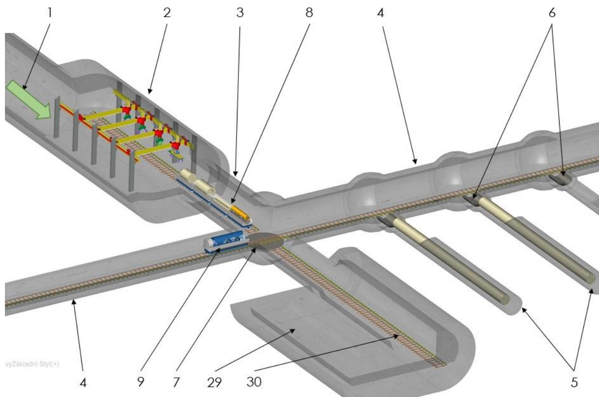
Obr. 68 – Koncepční model hlubinného úložiště
