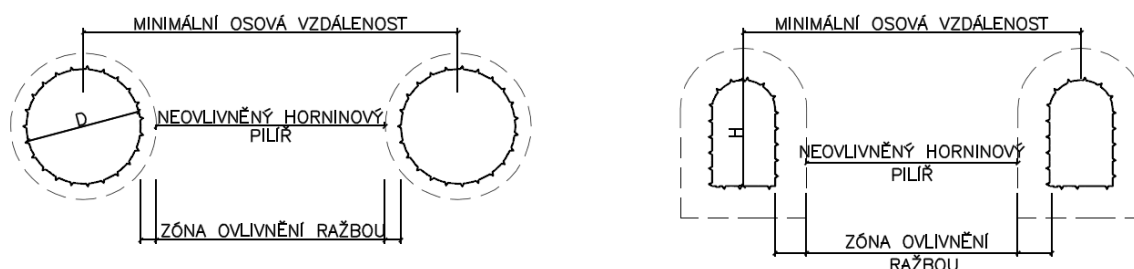
Obr. 56 – Princip stanovení minimální vzdálenosti mezi zav. chodbami / ukládacími vrty
