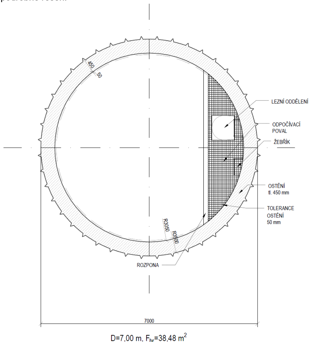
Obr. 75 – Příčný řez vtažnou jámou průměru 7,0 m
