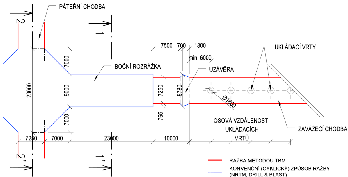
Obr. 78 – Půdorysné schéma ukládání – varianta D1
