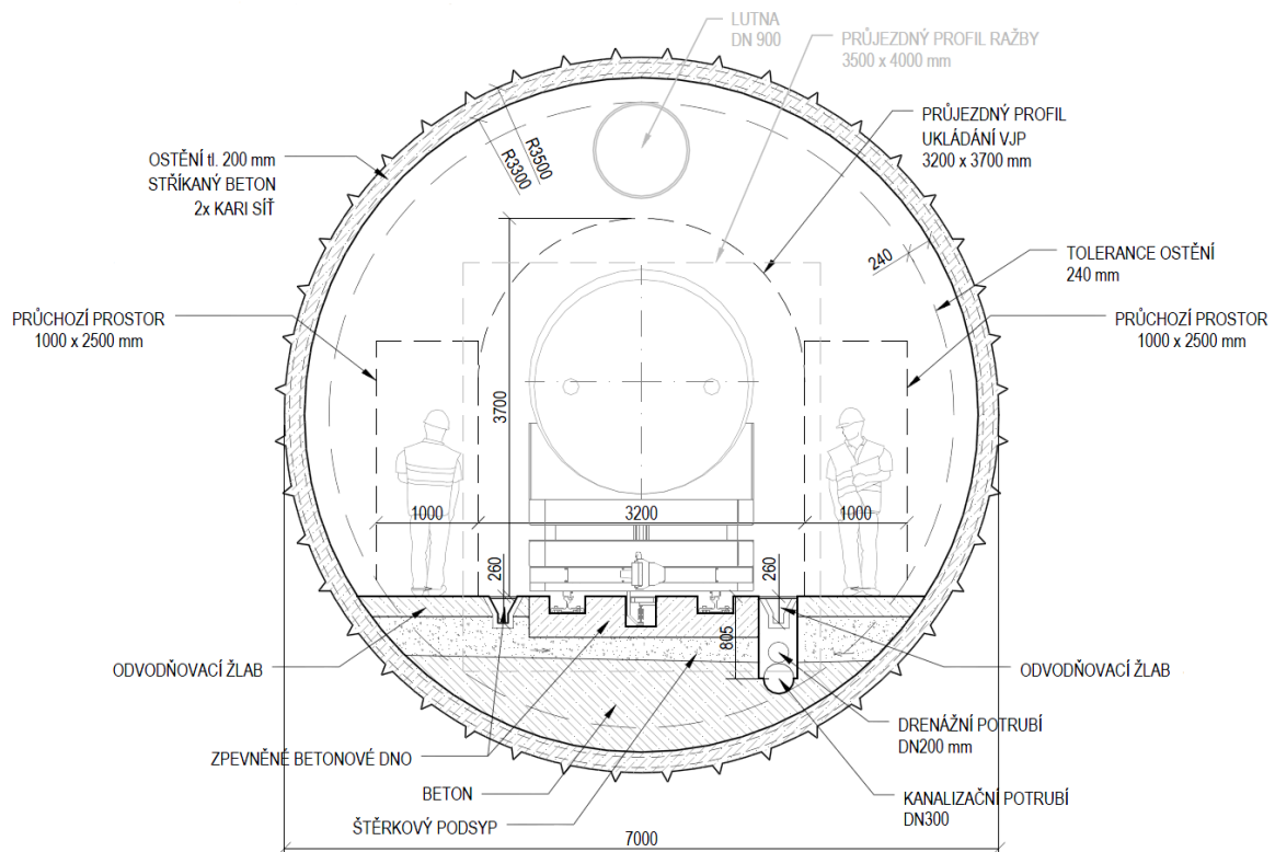
Obr. 76 – Příčný řez páteřní chodbou – D3
