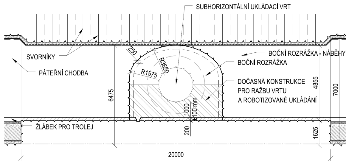
Obr. 85 – Příčný řez 2-2' boční rozrážkou – varianta D3
