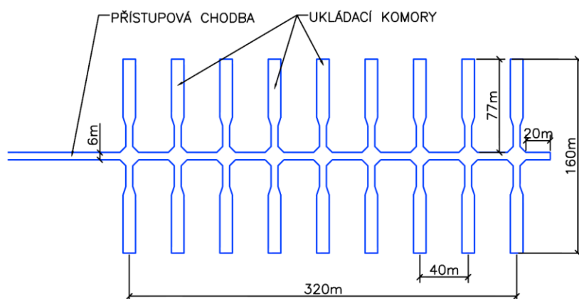
Obr. 89 - Schéma ukládání RAO
