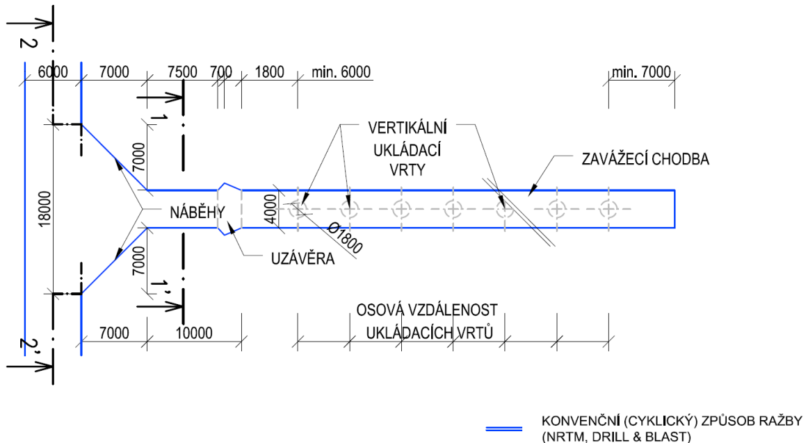
Obr. 80 – Půdorysné schéma ukládání – varianta D2
