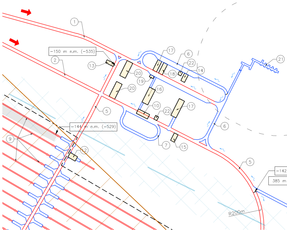
Obr. 58 – Schéma technického zázemí - D3
