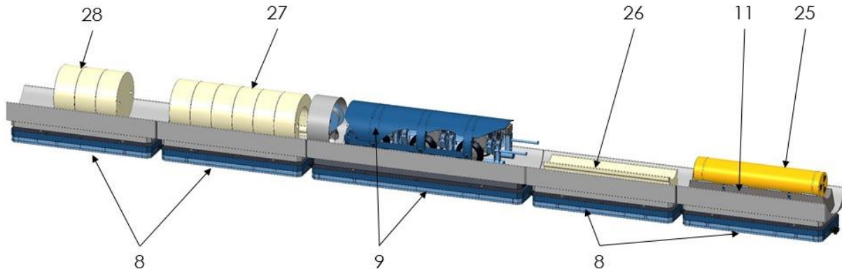
Obr. 69 – Souprava robotických vozů pro transport ÚOS a bentonitových prefabrikátů
