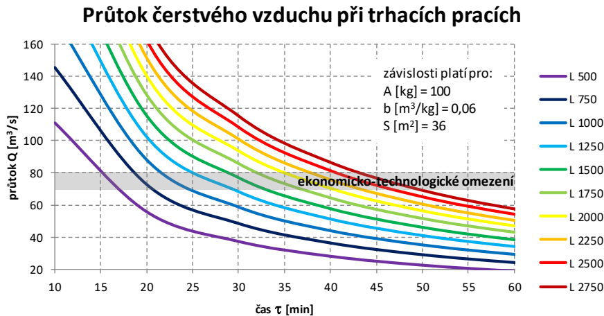
Obr. 64 – Závislost potřebného průtoku vzduchu při trhacích pracích na čase a délce ražby podle [56]
