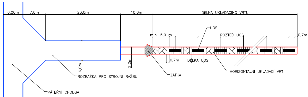
Obr. 55 – Schéma horizontálního ukládání, převládající konvenční ražba (D4)
