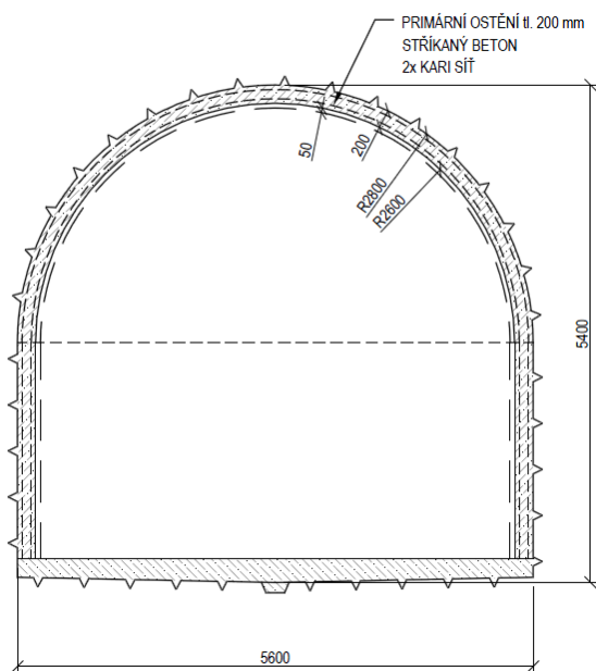
Obr. 91 – Příčný řez chodbou ústící do komory pro ukládání RAO
