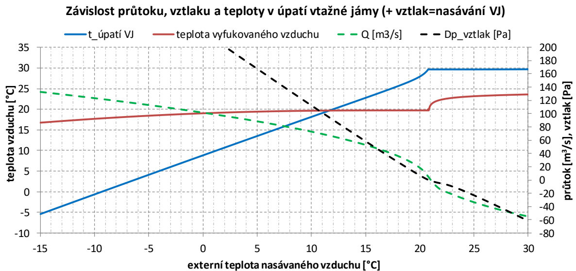
Obr. 61 – Průběhy teploty vzduchu v raženém díle, přirozeného vztlaku a průtoku v závislosti na externí teplotě.
