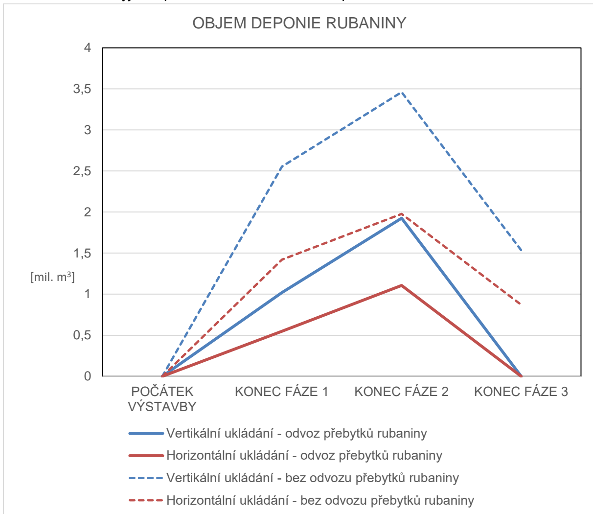
Obr. 96 – Předpokládaný objem deponie rubaniny na lokalitě Čertovka během budování, provozu a uzavírání HÚ
