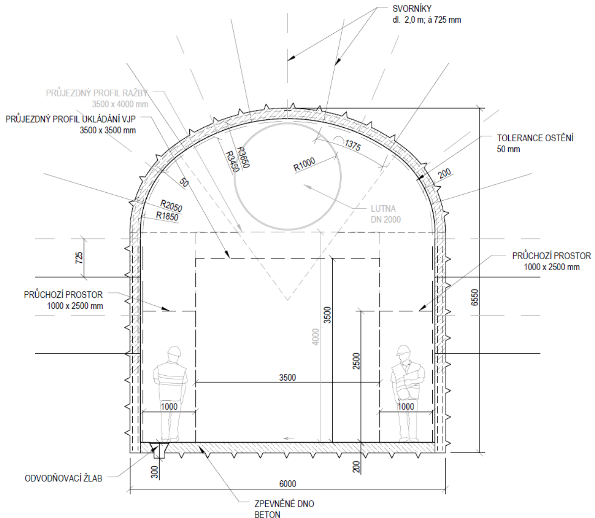
Obr. 74 – Příčný řez zavážecím tunelem, konvenční ražba, primární ostění – D2 a D4
