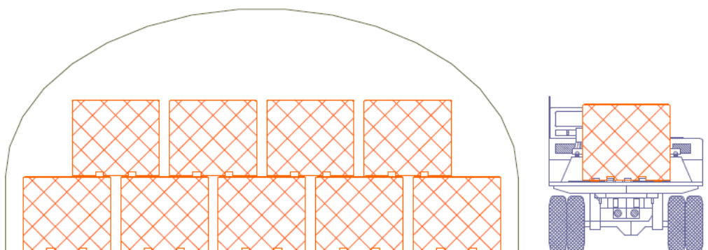
Obr. 70 – Ukládací komora RAO – příčný řez
