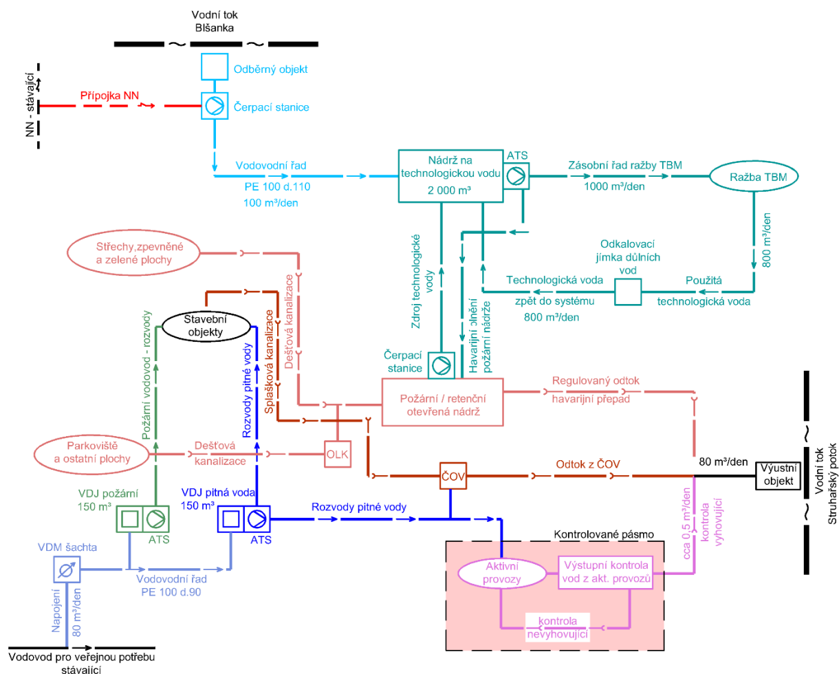
Obr. 95 – Schéma vodního hospodářství PA
