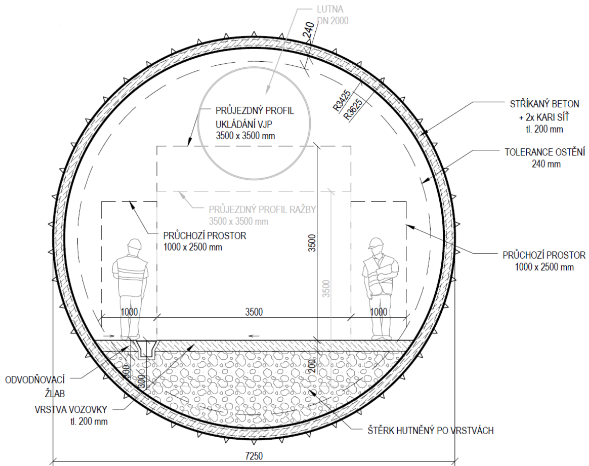
Obr. 72 – Příčný řez zavážecím a odtěžovacím tunelem – D1
