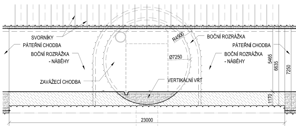
Obr. 79 – Podélný řez 2-2' s pohledem na boční rozrážku – varianta D1
