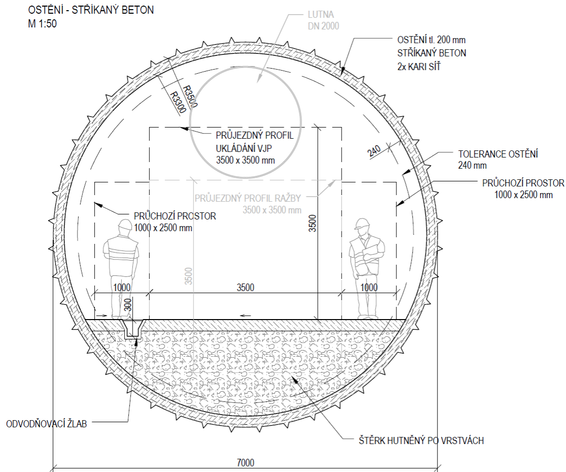
Obr. 73 – Příčný řez zavážecím a odtěžovacím tunelem – D3
