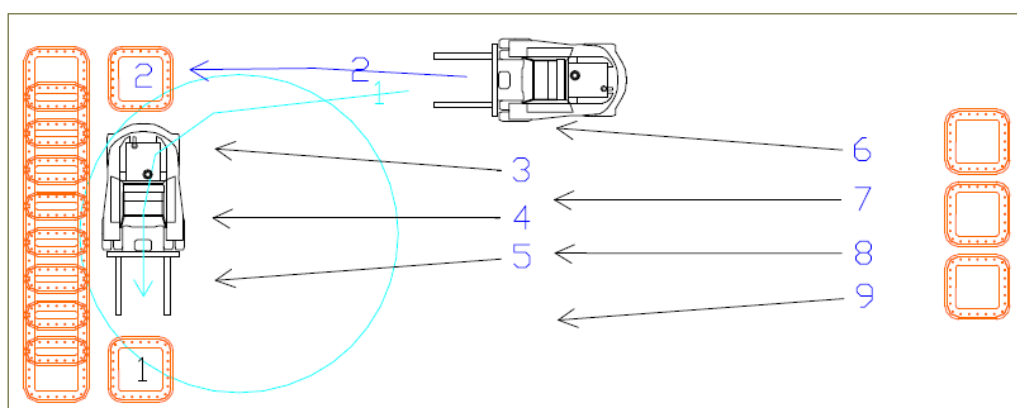
Obr. 71 – Ukládací komora RAO - půdorys
