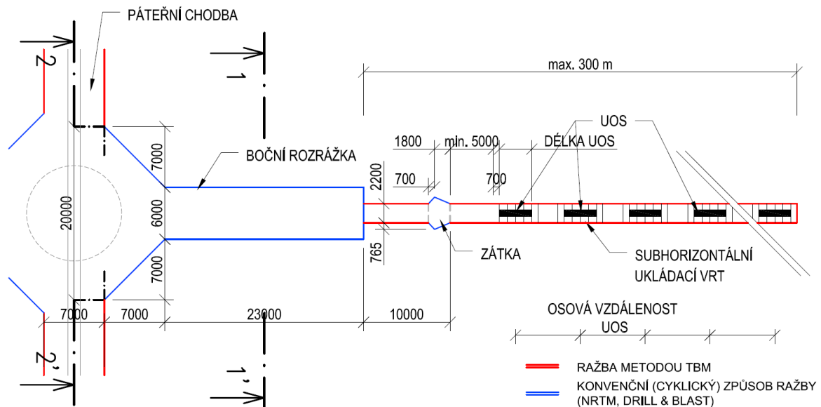
Obr. 84 – Půdorysné schéma ukládání – varianta D3
