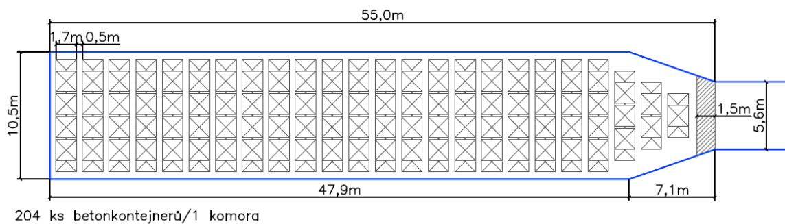
Obr. 88 - Ukládací komora RAO
