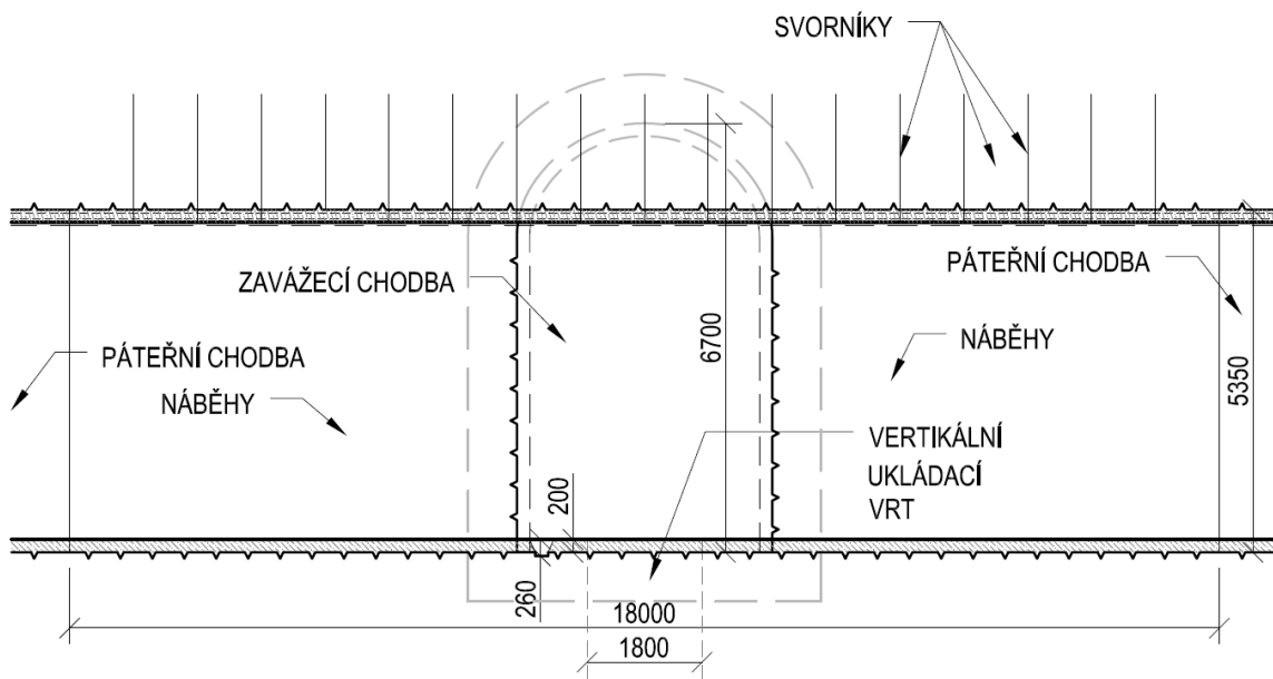
Obr. 81 – Příčný řez 2-2' ukládací chodbou – varianta D2
