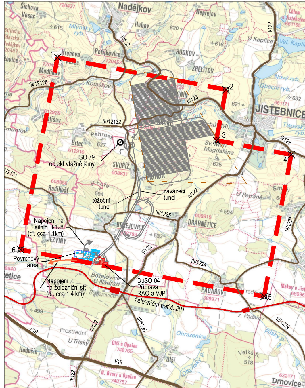
Dispoziční řešení D1 - vertikální ukládání, ražba TBM
