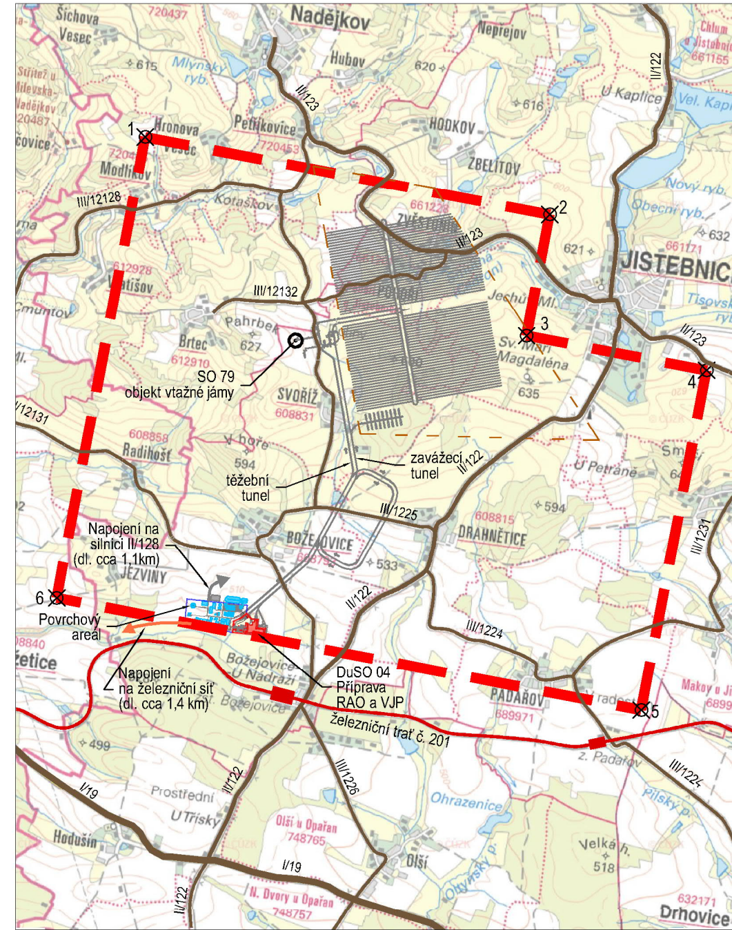
Dispoziční řešení D2 - vertikální ukládání, konvenční ražba
