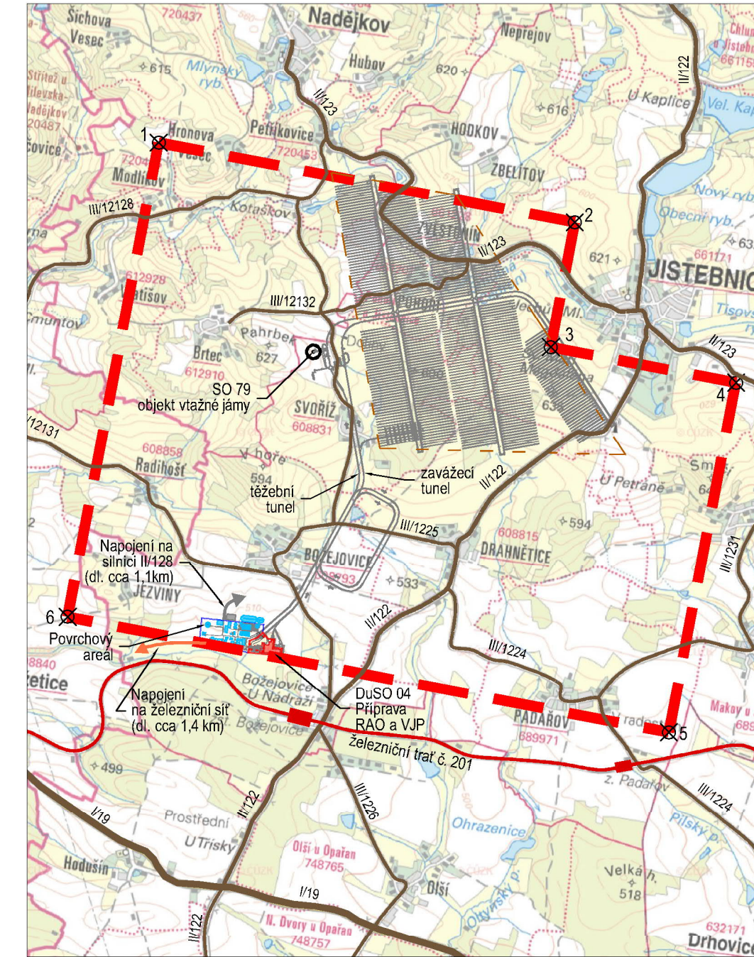
Dispoziční řešení D4 - horizontální ukládání, konvenční ražba
