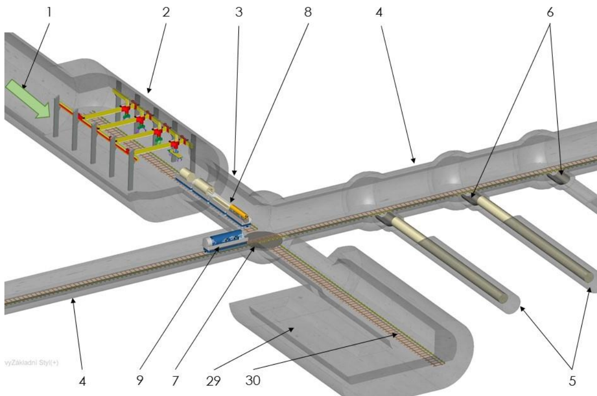
Obr. 61 – Koncepční model hlubinného úložiště
