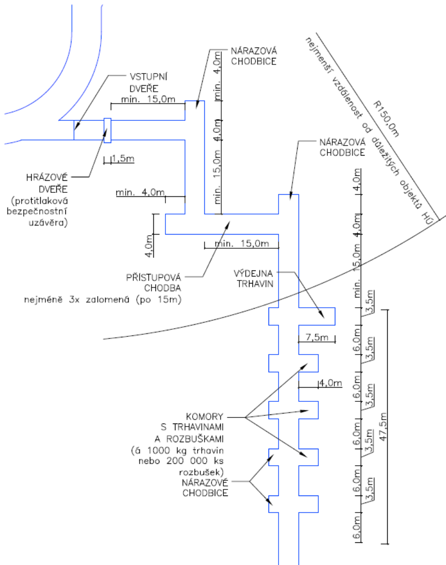
Obr. 85 – Schéma skladu výbušnin
