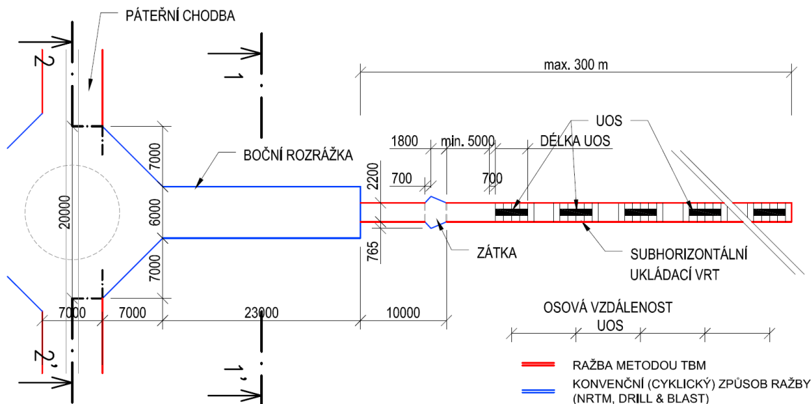
Obr. 77 – Půdorysné schéma ukládání – varianta D3
