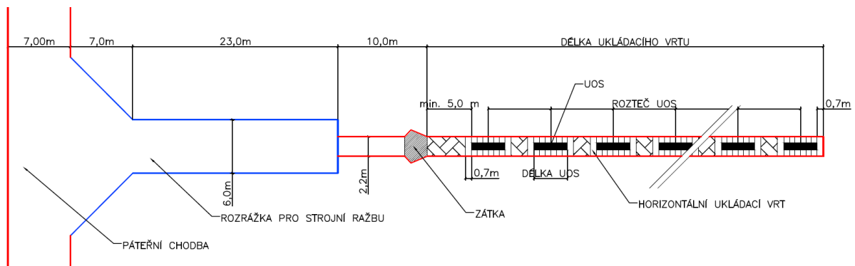
Obr. 48 – Schéma horizontálního ukládání, převládající mechanizovaná ražba (D3)
