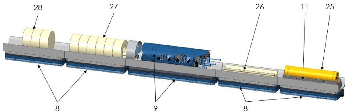
Obr. 62 – Souprava robotických vozů pro přepravu UOS a bentonitových prefabrikátů (převzato z [46])
