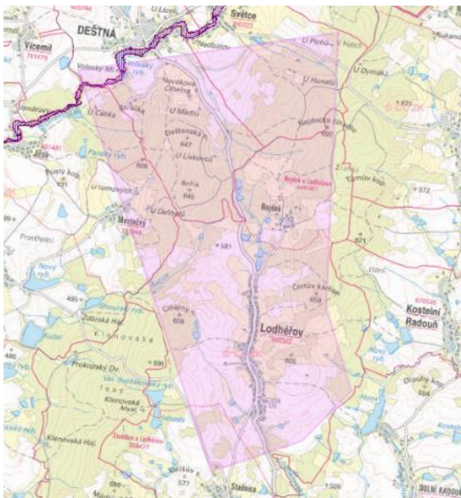
Obr. 13 – Záplavová území Q100
