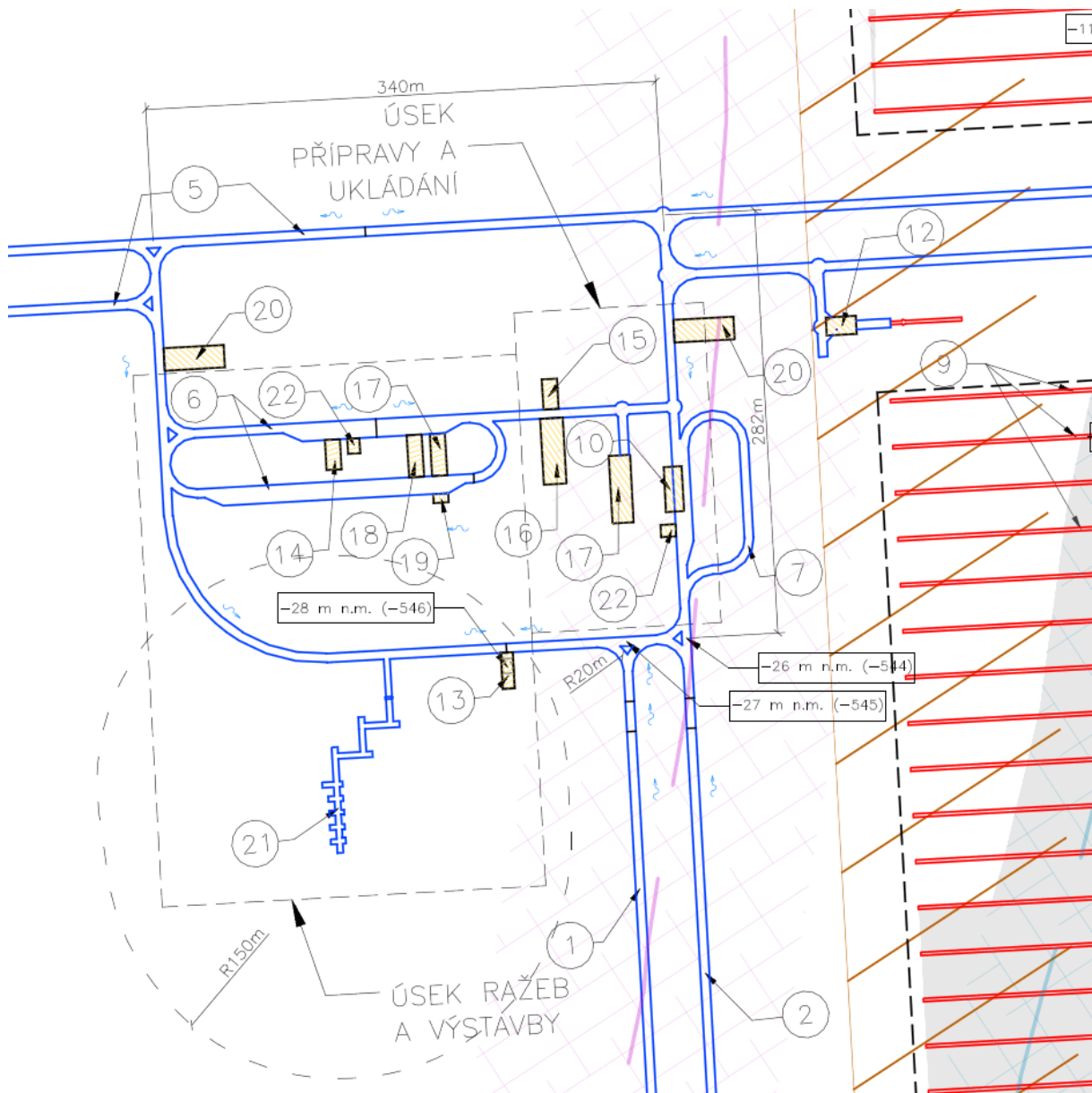
Obr. 54 – Schéma technického zázemí - D4
