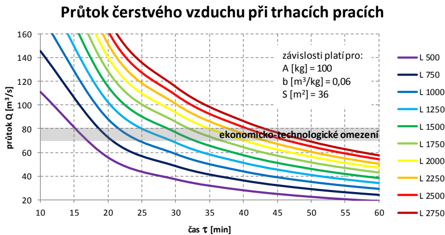
Obr. 56 – Závislost potřebného průtoku vzduchu při trhacích pracích na čase a délce ražby podle [43]
