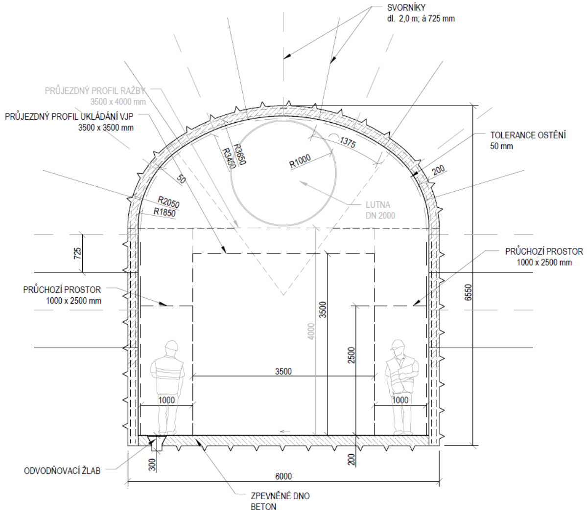
Obr. 67 – Příčný řez zavážecím tunelem, konvenční ražba, primární ostění – D2 a D4
