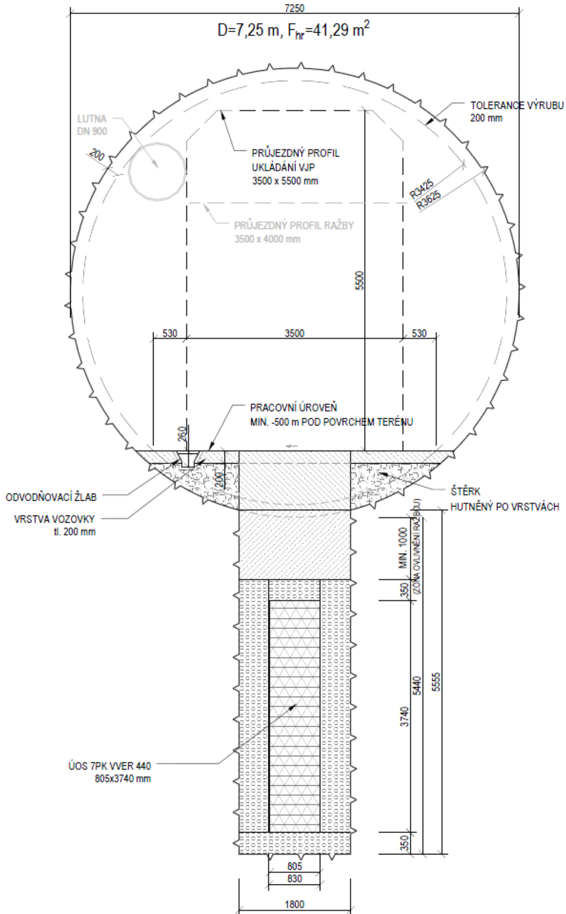
Obr. 75 – Vertikální uložení UOS (VVER 440) z ukládací chodby ražené TBM - D1
