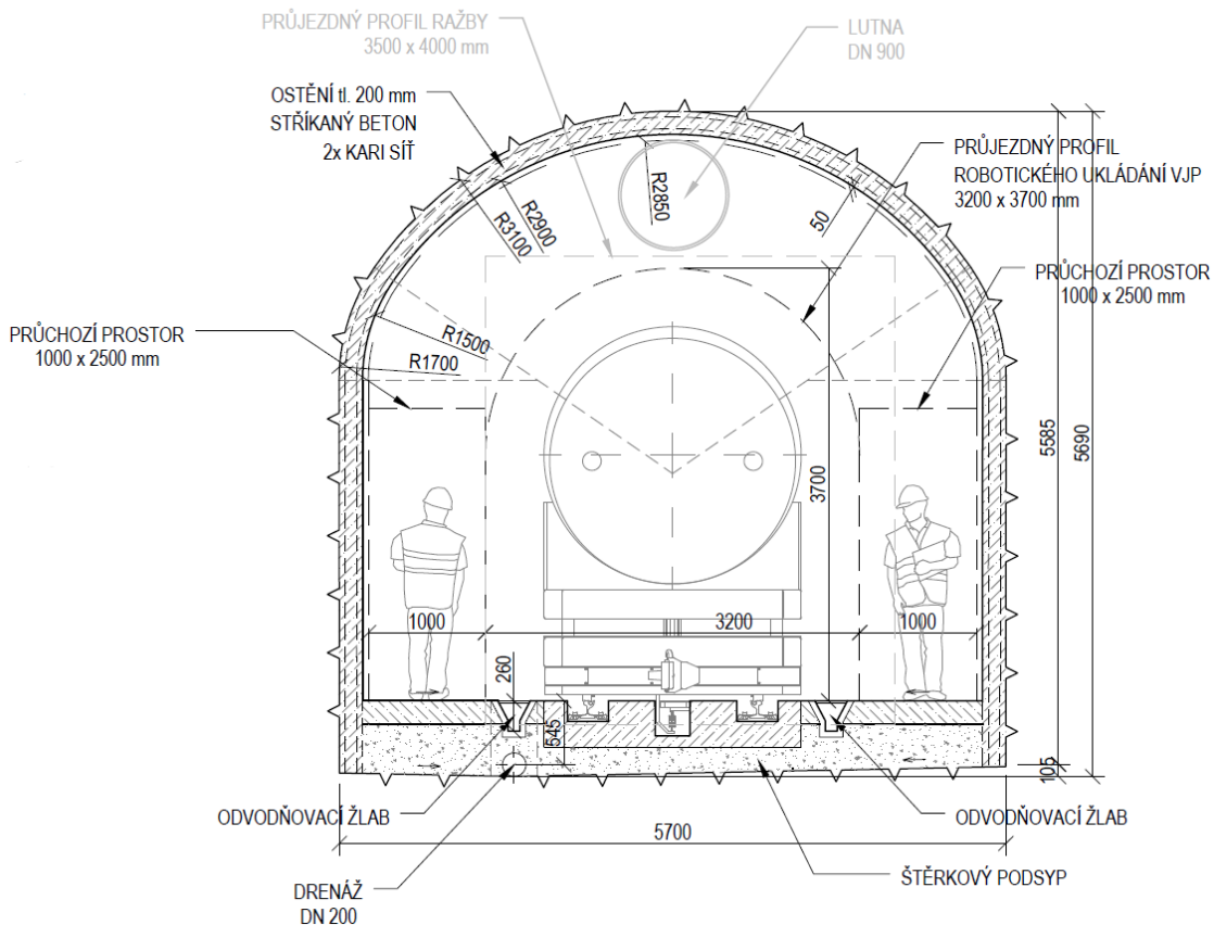
Obr. 70 – Příčný řez páteřní chodbou – D4
