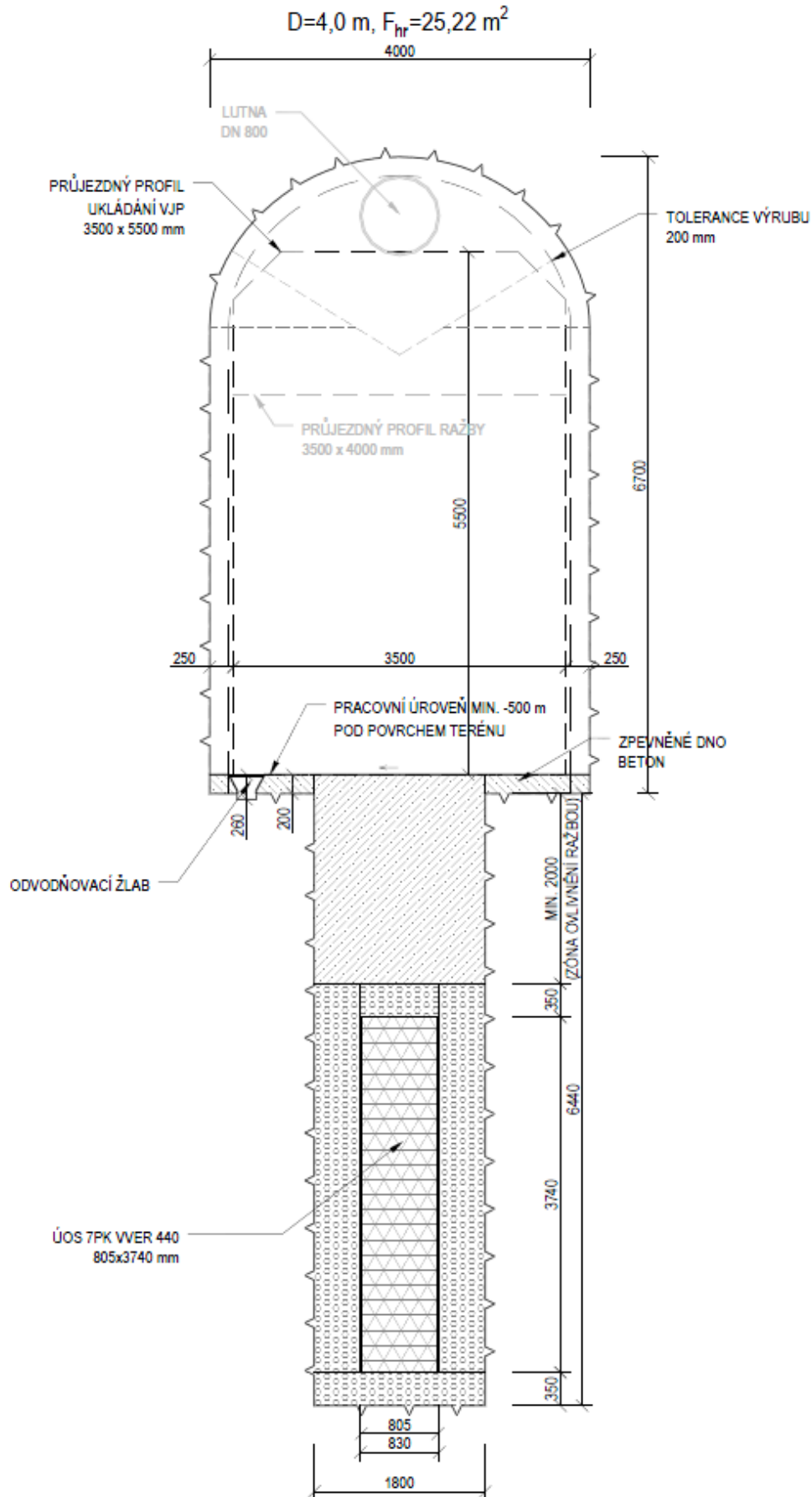
Obr. 76 - Vertikální uložení UOS (VVER 440) z ukládací chodby ražené konvenčně - D2
