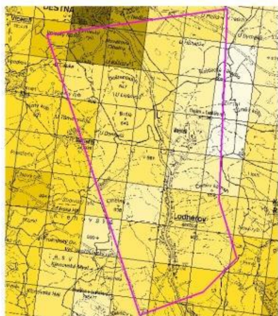
Obr. 5 – PM 10 průměrná roční koncentrace - pětileté průměry 2011-2015 ve čtvercové síti 1km x 1km
