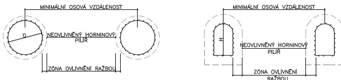
Obr. 50 – Princip stanovení minimální vzdálenosti mezi zav. chodbami / ukládacími vrty
