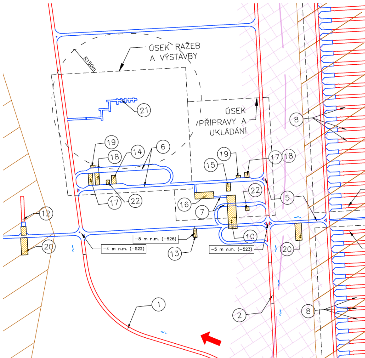
Obr. 51 - Schéma technického zázemí - D1
