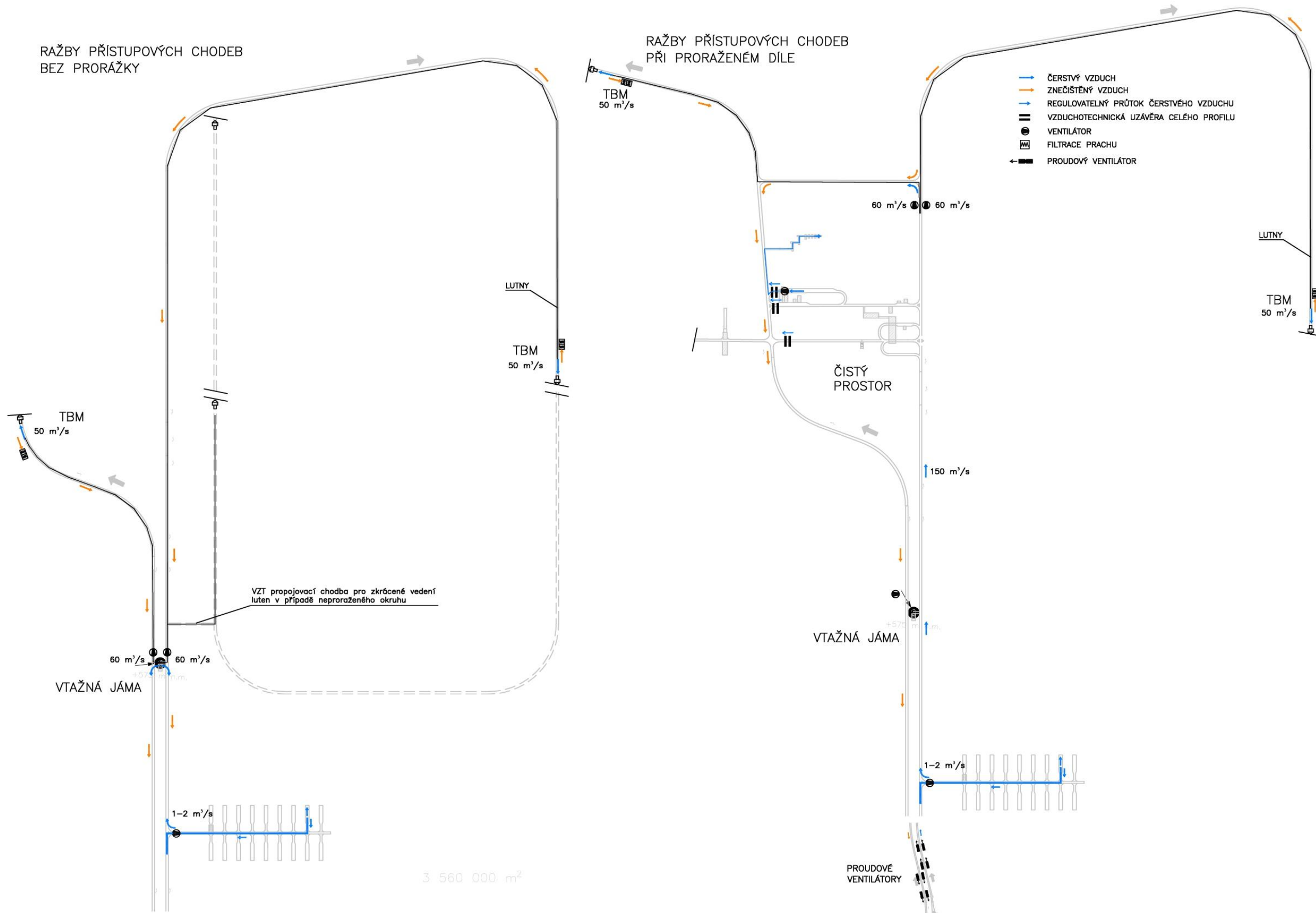
Obr. 57 – Schéma větrání při ražbě přístupových chodeb pomocí TBM
