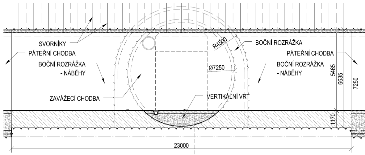
Obr. 72 – Podélný řez 2-2' s pohledem na boční rozrážku – varianta D1
