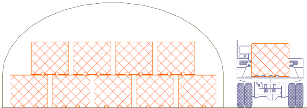
Obr. 63 – Ukládací komora RAO – příčný řez
