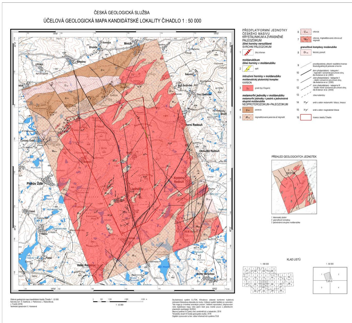
Obr. 24 – Geologická mapa lokality Čihadlo
