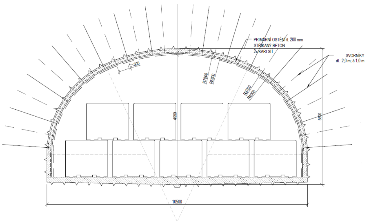
Obr. 83 – Příčný řez komorou pro ukládání RAO
