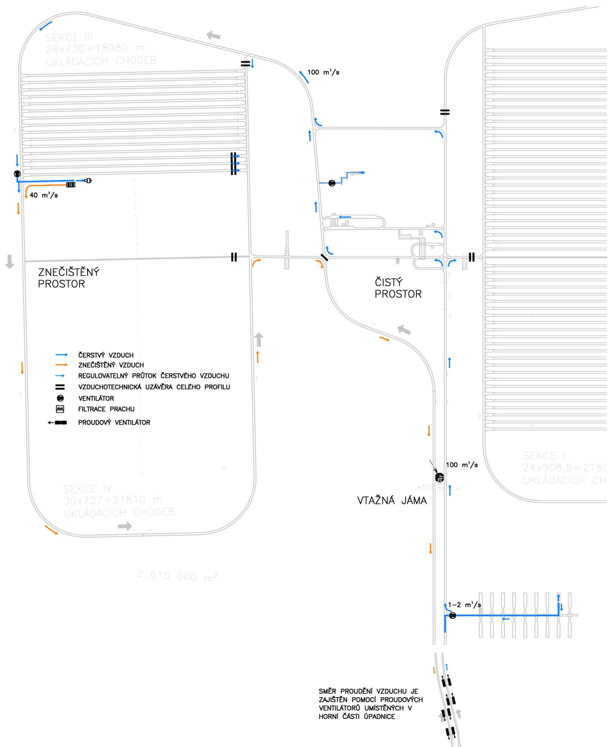
Obr. 60 – Schéma větrání HÚ při ražbách zavázečních chodeb pomocí TBM a zavážení VJP do úložiště v sekci III. Sekce I a II jsou zavezeny a trvale uzavřeny.
