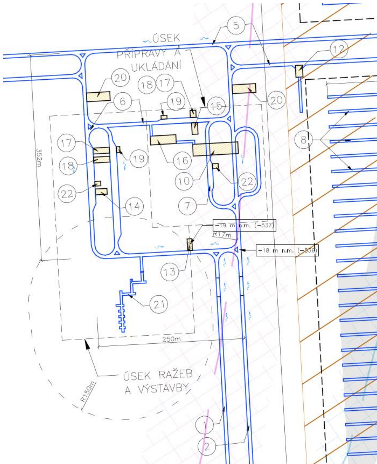
Obr. 53 – Schéma technického zázemí - D2
