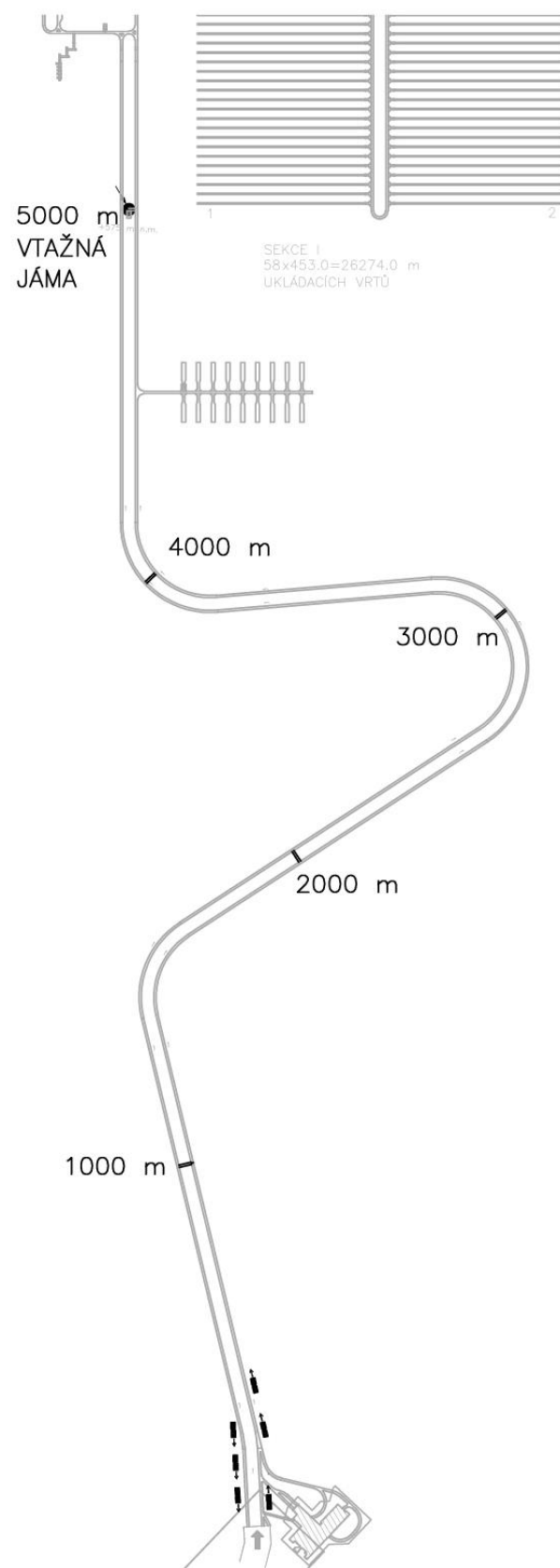
Obr. 55 – Schéma větrání při konvenční ražbě úpadních tunelů
