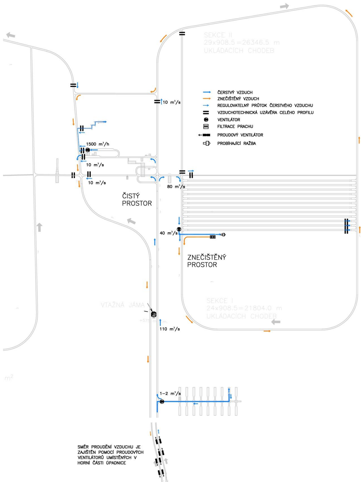
Obr. 59 – Schéma větrání HÚ při ražbách pomocí TBM zavázečních chodeb a zavázení VJP do úložiště v sekce I
