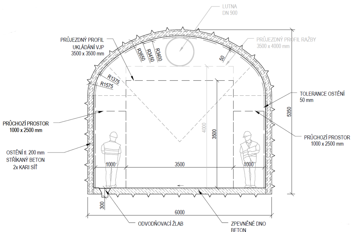
Obr. 69 – Příčný řez páteřní chodbou – D2
