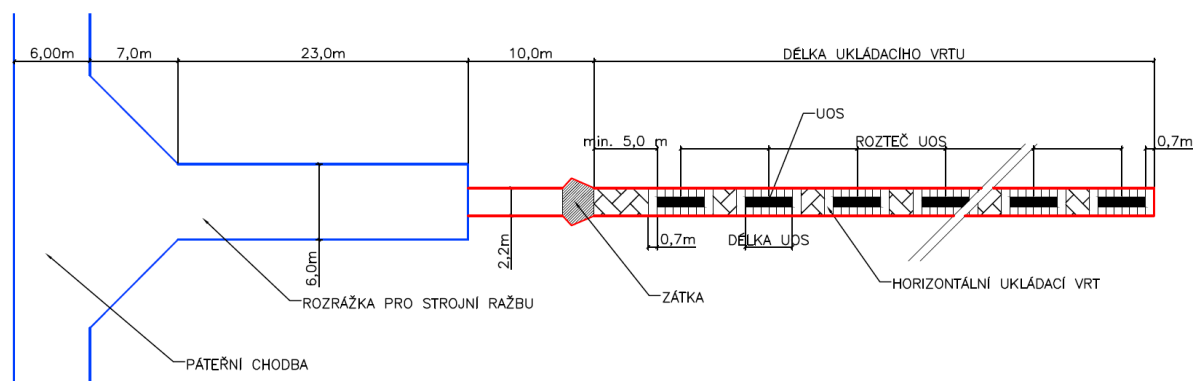
Obr. 49 – Schéma horizontálního ukládání, převládající konvenční ražba (D4)
