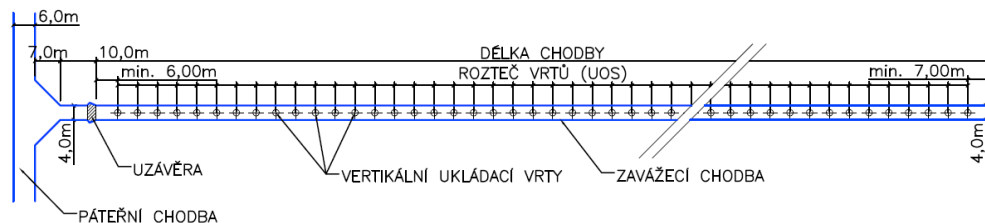
Obr. 47 – Schéma vertikálního ukládání, převládající konvenční ražba (D2)
