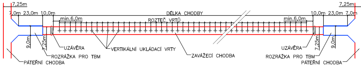
Obr. 46 – Schéma vertikálního ukládání, převládající mechanizovaná ražba (D1)
