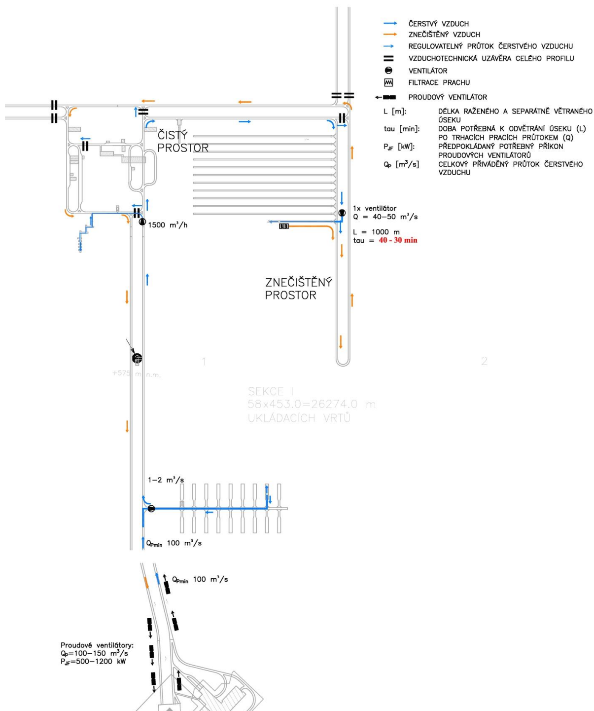
Obr. 58 – Schéma větrání HÚ při ražbách zavázečních chodeb konvenční metodou a zavážení VJP do úložiště v sekci I.
